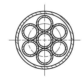
支柱断面詳細図 S=1:3
