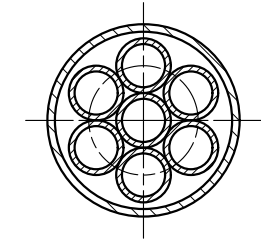
支柱断面詳細図 S=1:3
