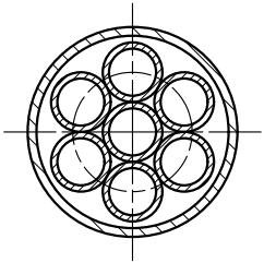
支柱断面詳細図 S=1:3
