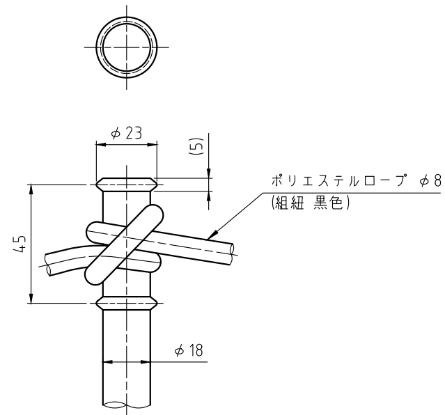
支柱頂部詳細図 S=1:2
