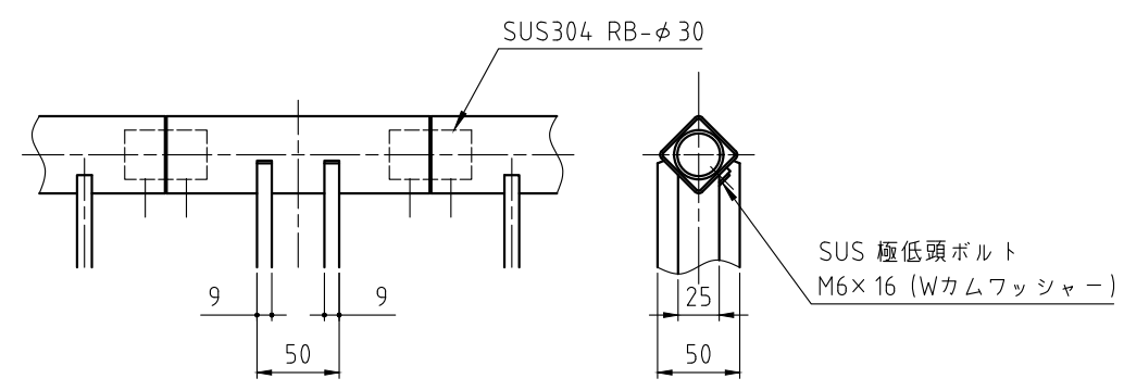
支柱頂部詳細図 S=1:5
