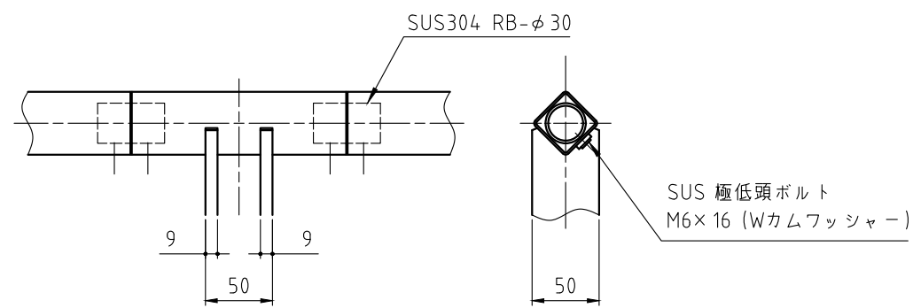
支柱頂部詳細図 S=1:5
