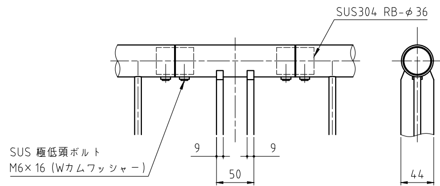
支柱頂部詳細図 S=1:5
