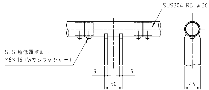
支柱頂部詳細図 S=1:5
