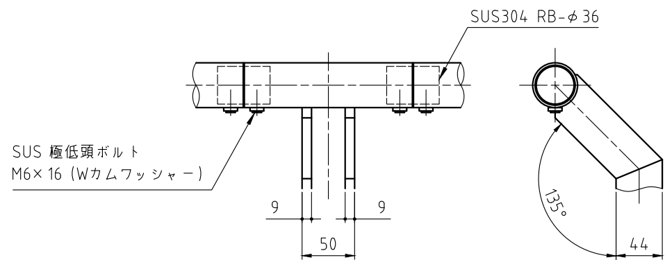
支柱頂部詳細図 S=1:5
