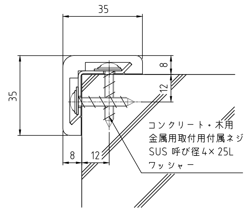
取付断面詳細図 S=1:1
