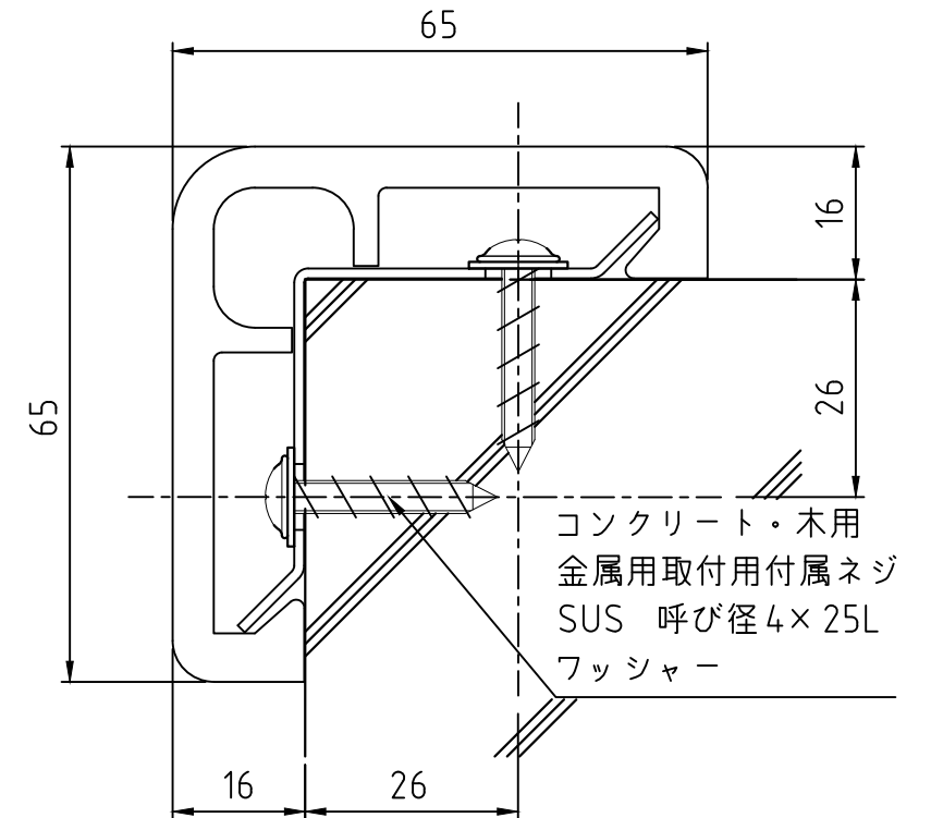
取付断面詳細図 S=1:1
