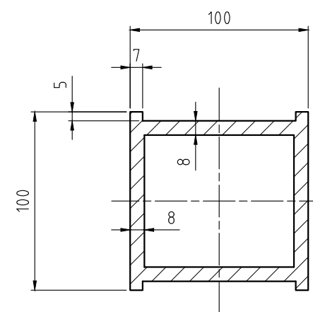
A-A 断面詳細図 S=1:3
