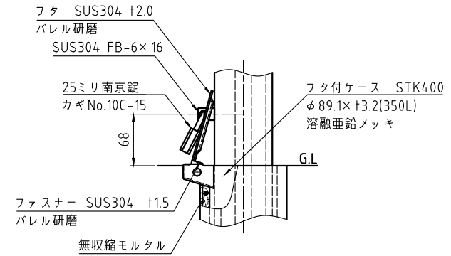
施錠部詳細図 S=1:5
