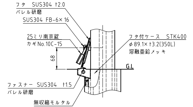
施錠部詳細図 S=1:5
