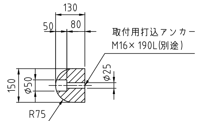
A-A断面図
