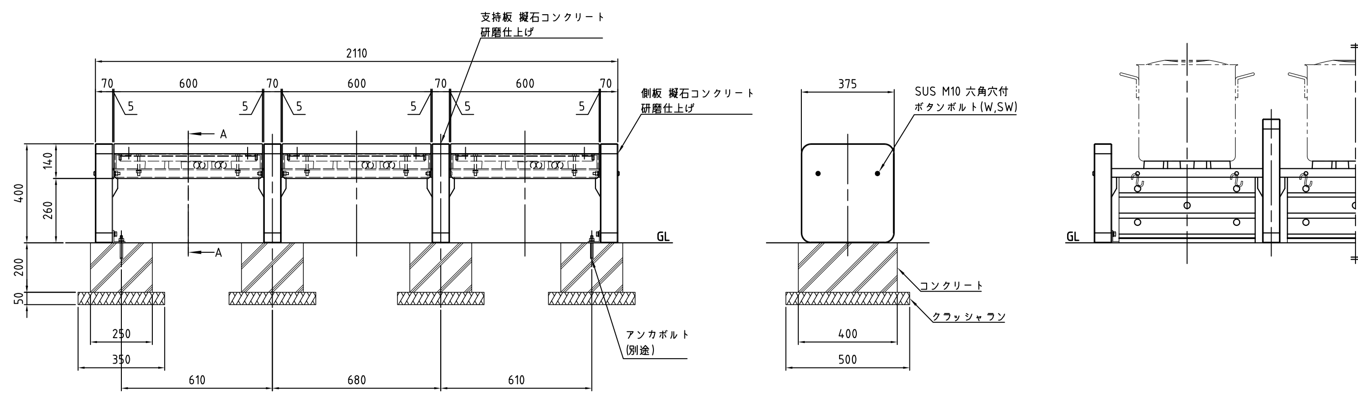
A-A S=1:5
